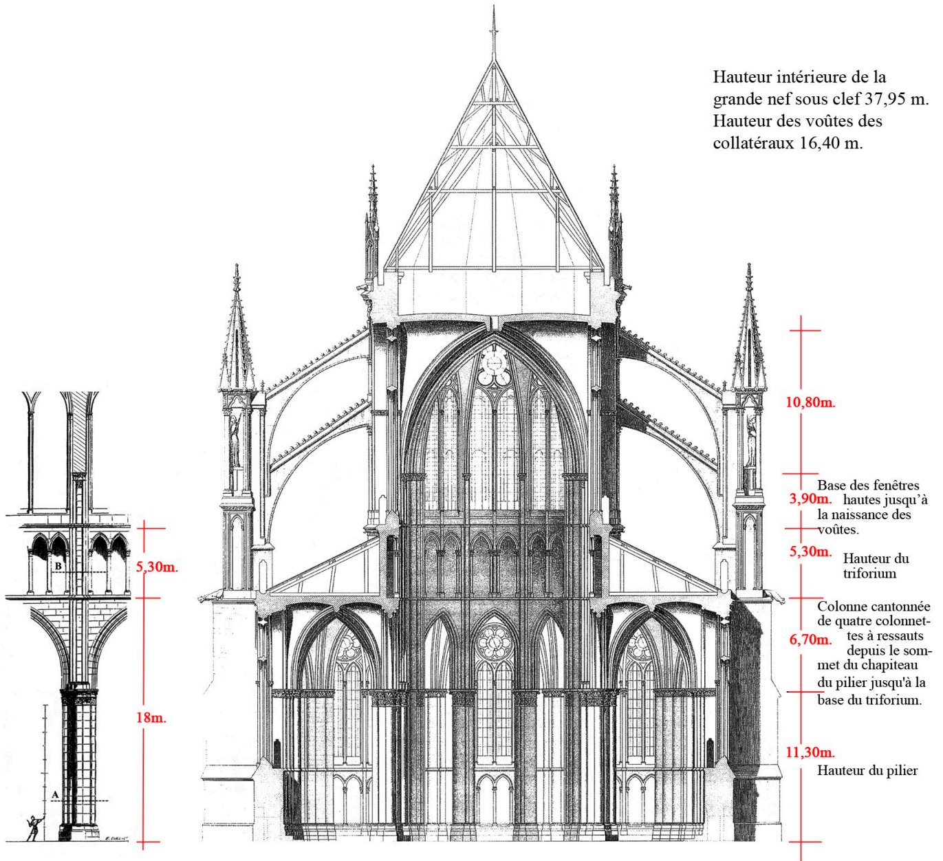
Elévation et sections de pilier, d'après un dessin de Viollet-le-Duc
